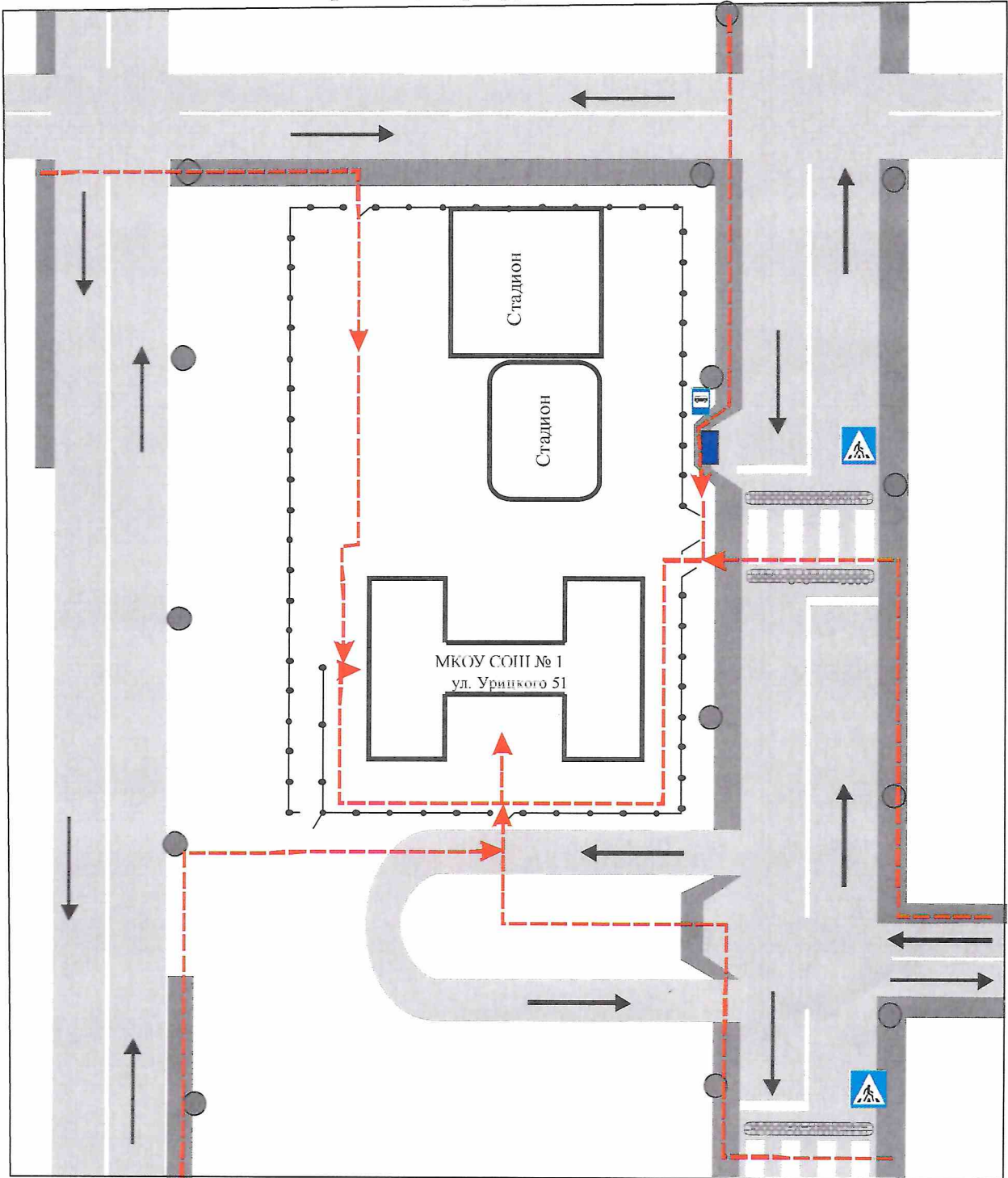
Схема организации дорожного движения в непосредственной близости от образовательного учреждения с размещением соответствующих технических средств, маршруты движения детей.
